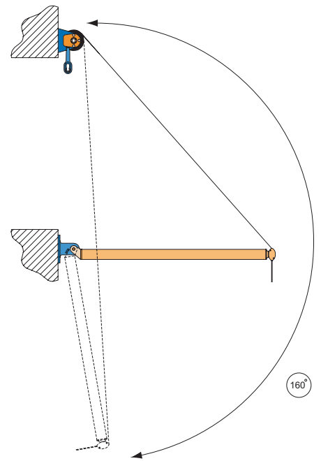
Widok z boku - markiza otwarta Powyżej kąta 90° dopłata za tkaninę
