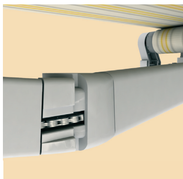
Ramię z łańcuchem
