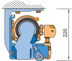
Montaż do sufitu
