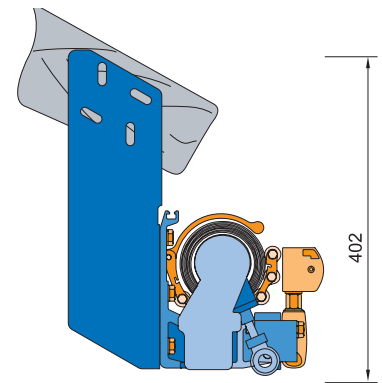
Montaż do krokwi dachowej
