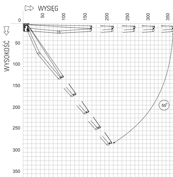
Zakres regulacji kąta nachylenia markizy
